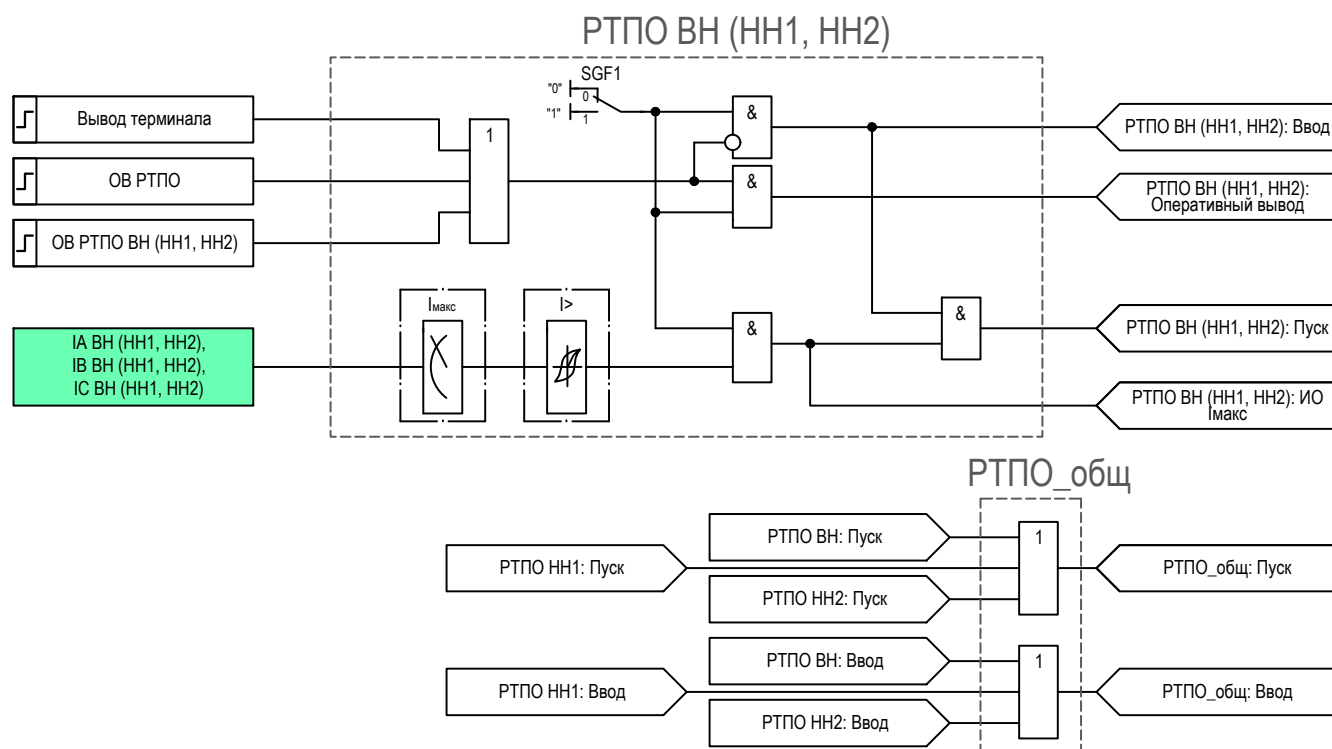
Рисунок 2.15 – Функциональная схема логики РТПО
