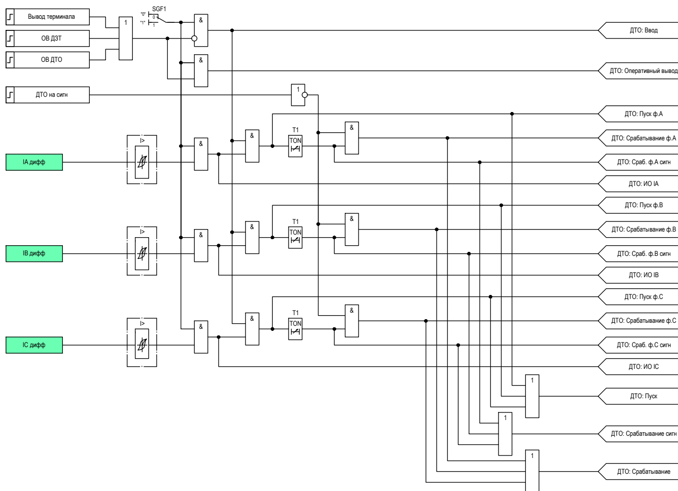
Рисунок 2.4 – Функциональная схема логики ДТО
