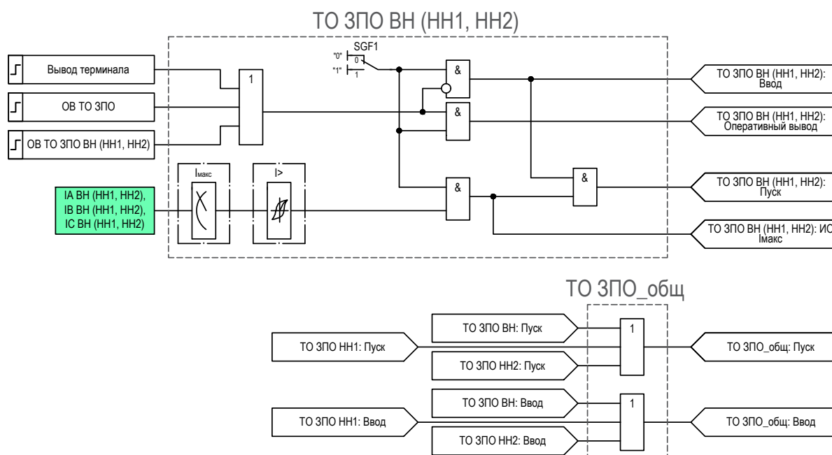
Рисунок 2.13 – Функциональная схема логики ТО ЗПО
