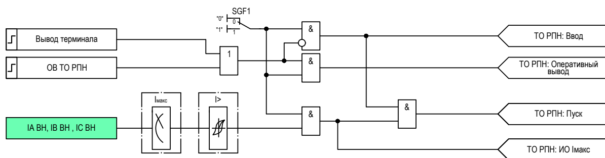
Рисунок 2.17 – Функциональная схема логики ТО РПН
